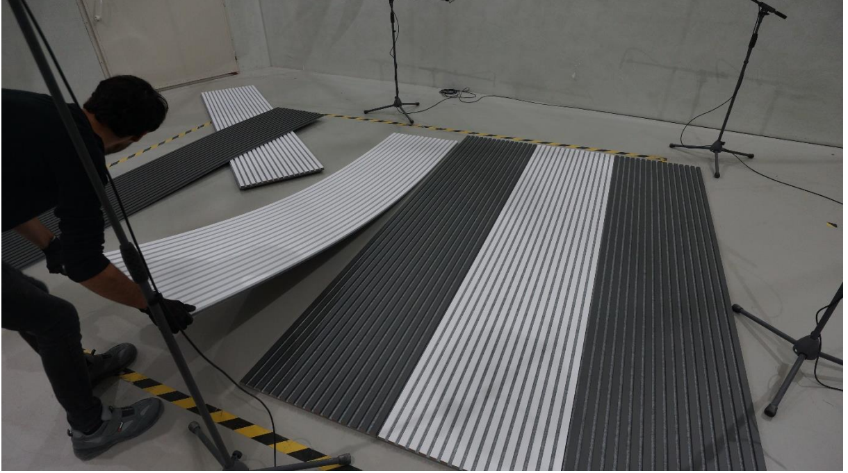
Şekil 5.2 Numunenin Ölçüme Hazırlık Süreci
